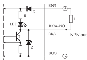
NPN output
