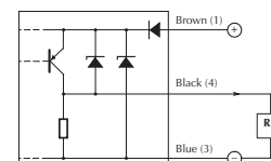
PNP output
