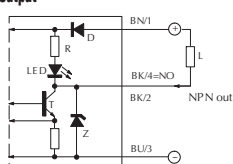
NPN Output
