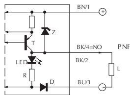
PNP output
