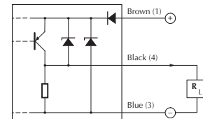
PNP Output
