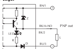
PNP Output
