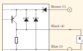
PNP output
