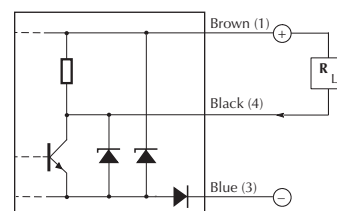
NPN Output
